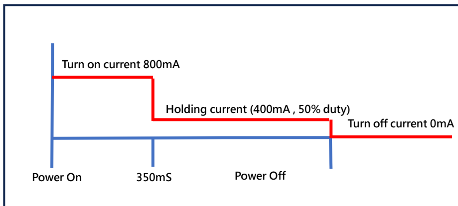
拓扑示例（50%占空比）
